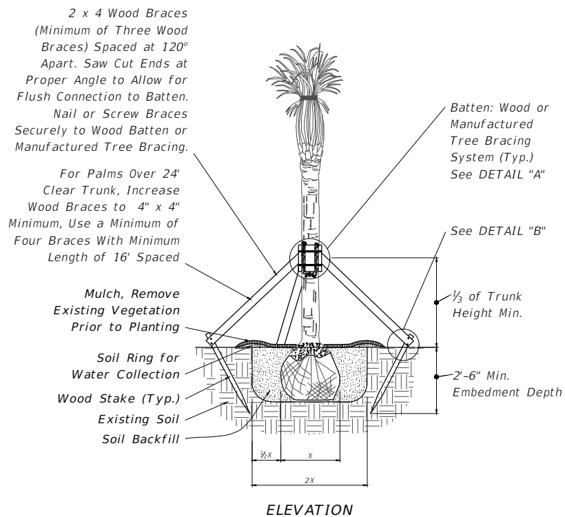
ELEVATION
